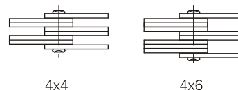
鏈板組合 Plate lacing
