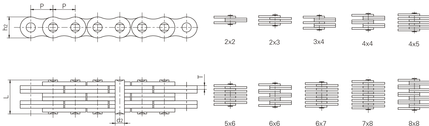
鏈板組合 Plate lacing
